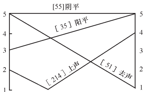
图 1-9 普通话调值示意图
