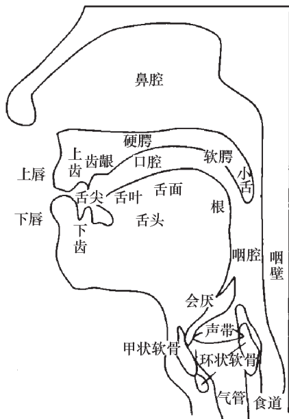
图 1-1 发音器官切面示意图
