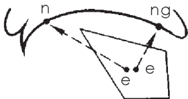
图 1-7 en 与 eng 发音示意图
