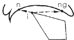
图 1-8 in 与 ing 发音示意图
