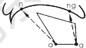
图 1-6 an 与 ang 发音示意图
