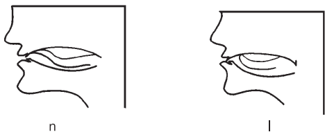
图 1-3 n、l 发音示意图
