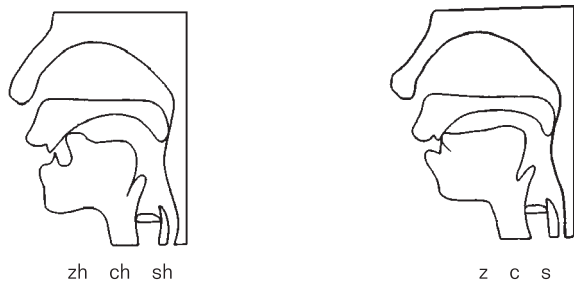
图 1-2 zh、ch、sh 和 z、c、s 发音示意图
