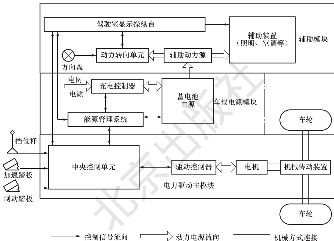
图 2-1-15 电力驱动控制系统的组成与工作原理
