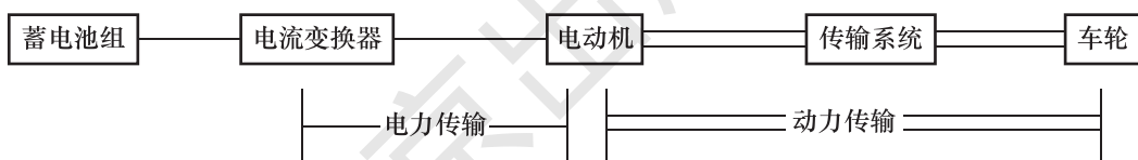
图 2-1-13 单一蓄电池作为动力源的纯电动汽车的电力和动力传输系统
