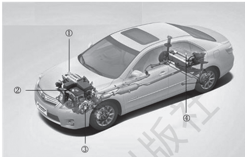
图 2-1-21 丰田凯美瑞混合动力汽车动力总成组成示意图
