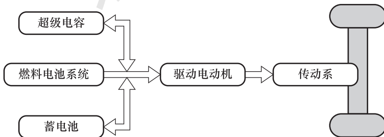
图 2-1-25 燃料电池与辅助蓄电池和超级电容联合驱动的电动汽车的动力系统结构
