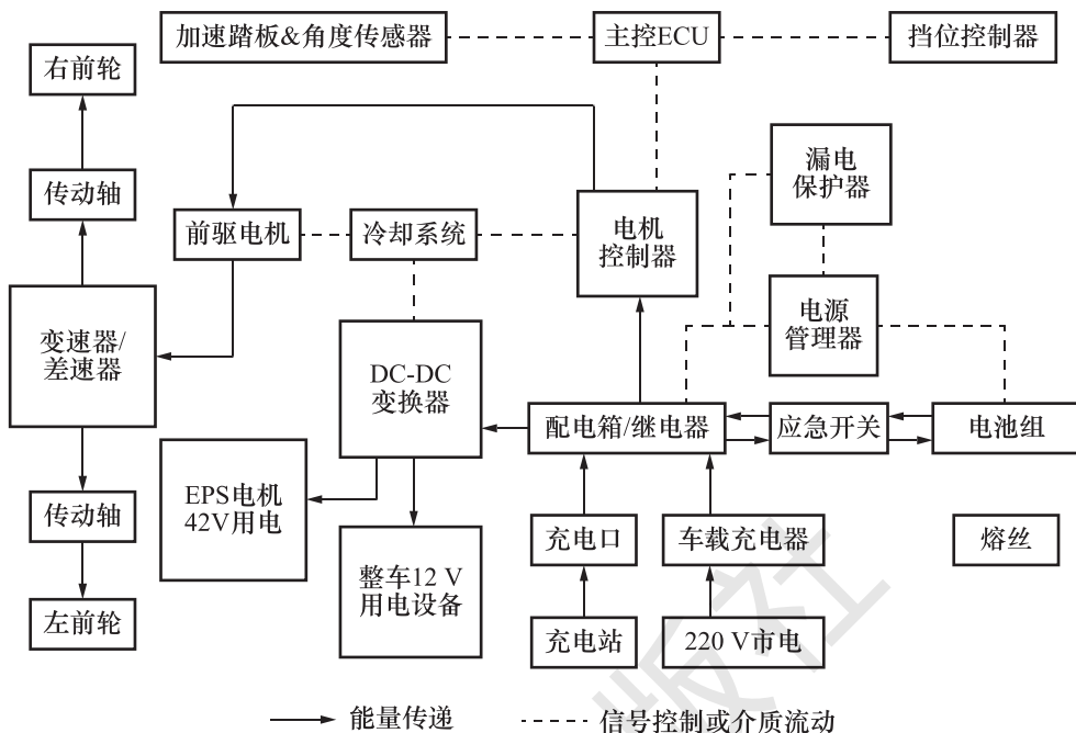
图 2-1-17 比亚迪 e6 工作原理框图
