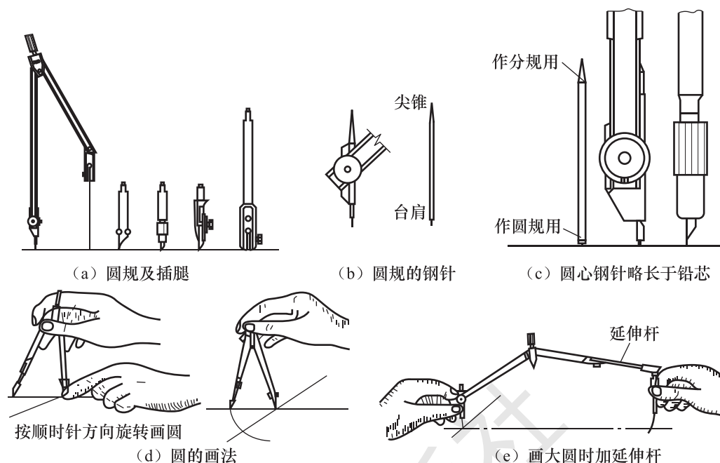
图 1-7 圆规的用法
