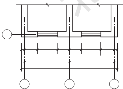
图 1-22 尺寸的排列
