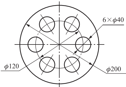
图 1-38 相同要素尺寸标注方法
