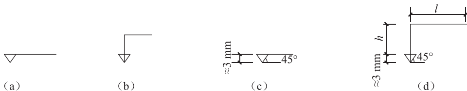
图 1-42 标高符号
