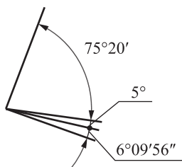
图 1-28 角度标注方法
