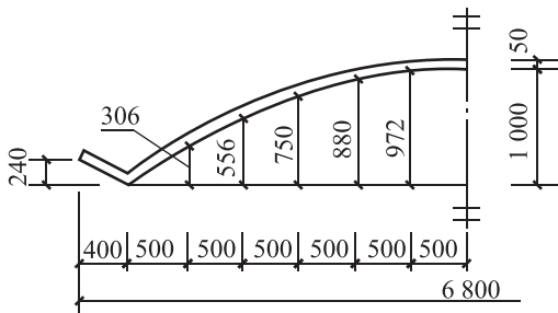
图 1-34 坐标法标注曲线尺寸
