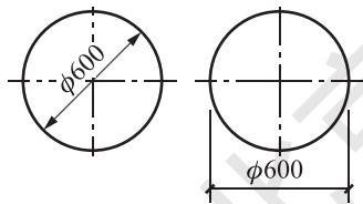
图 1-26 圆直径的标注方法
