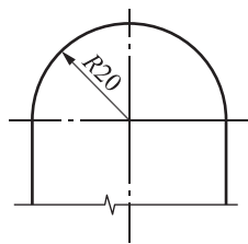
图 1-23 半径标注方法
