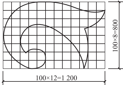
图 1-35 网格法标注曲线尺寸
