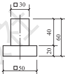
图 1-32 正方形标注方法
