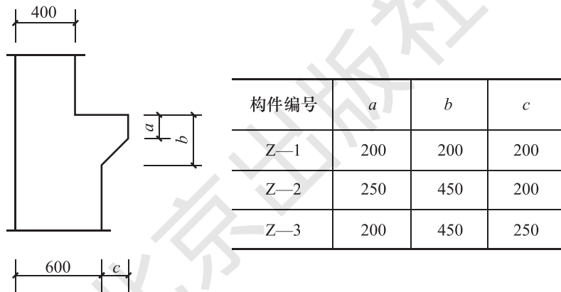
图 1-41 相似构配件尺寸表格式标注方法
