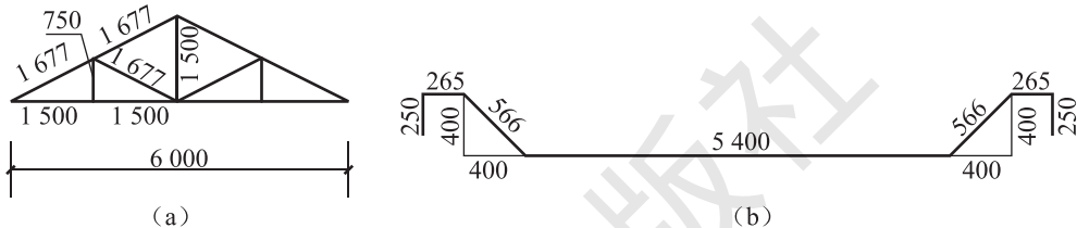
图 1-36 单线图尺寸标注方法
