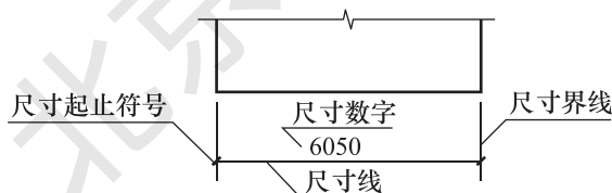
图 1-16 尺寸的组成
