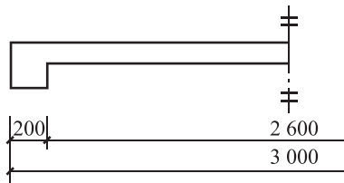
图 1-39 对称构配件尺寸标注方法
