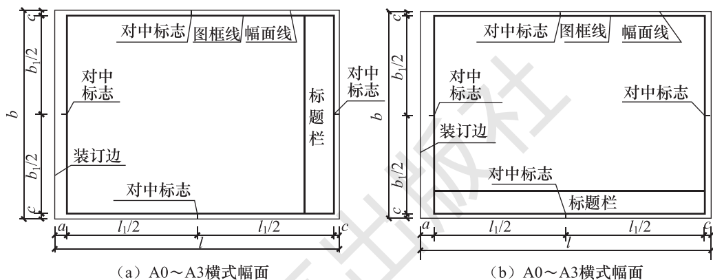
图 1-11 横式幅面
