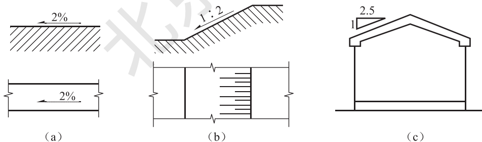
图 1-33 坡度标注方法
