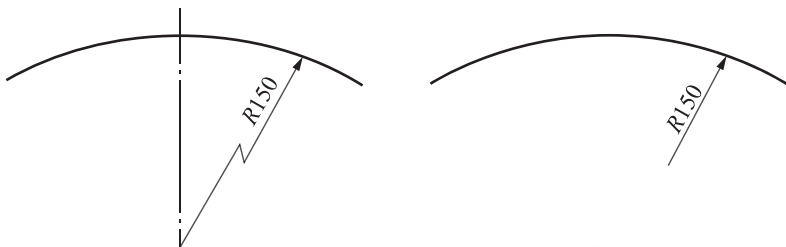
图 1-25 大圆弧半径的标注方法
