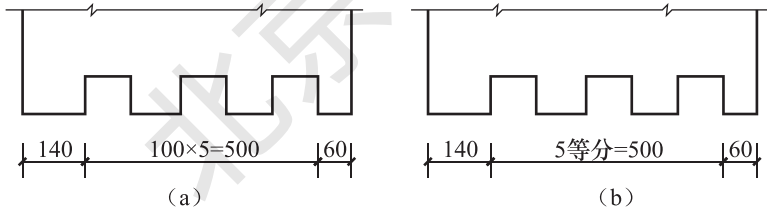
图 1-37 等长尺寸简化标注方法
