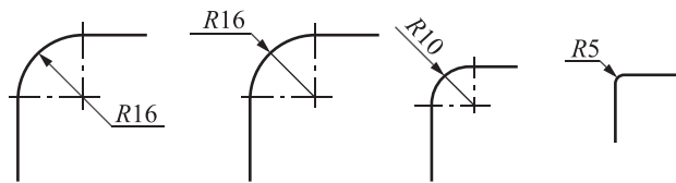
图 1-24 小圆弧半径的标注方法
