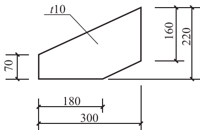
图 1-31 薄板厚度标注方法
