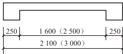
图 1-40 相似构配件尺寸标注方法
