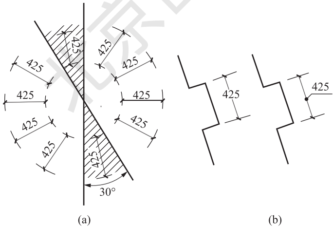
图 1-19 尺寸数字的注写方向
