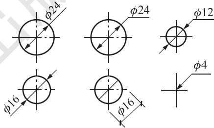
图 1-27 小圆直径的标注方法
