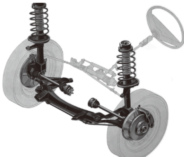
图 1-2-1 悬架系
