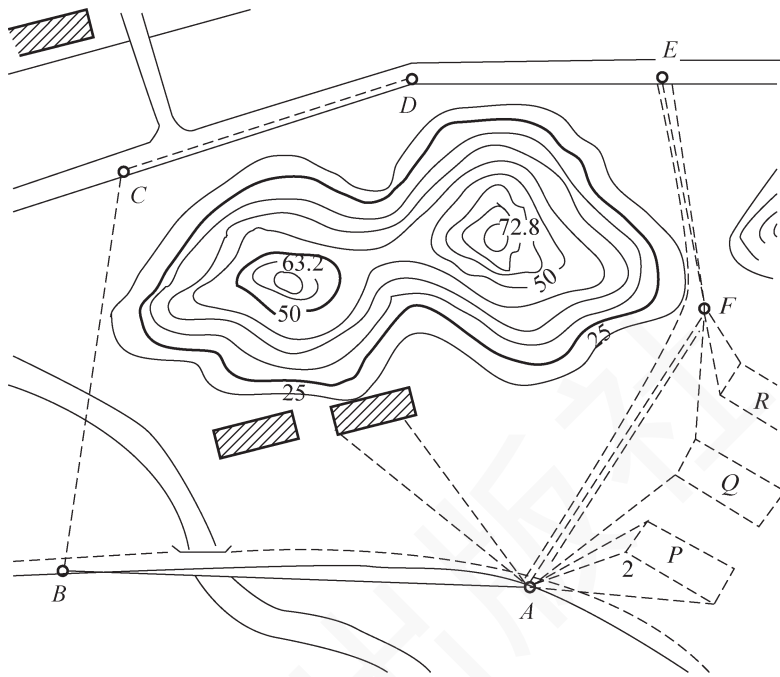
图 1-11 测量工作基本原则
