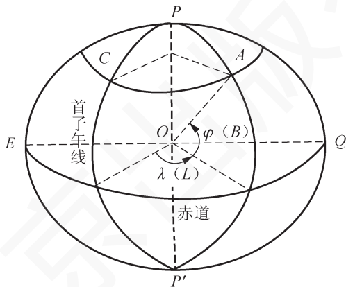
图 1-2 地理坐标
