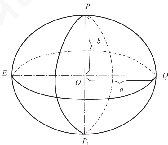
图 1-1 旋转椭球体
